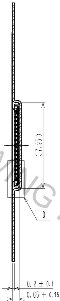
C-C (5:1)
