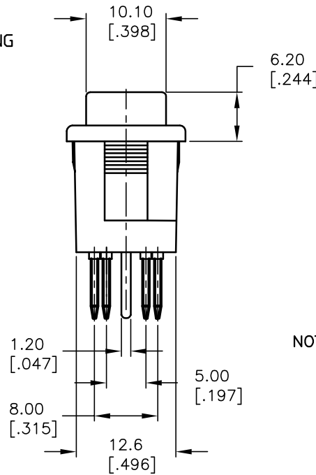
CIRCUIT: DPST
